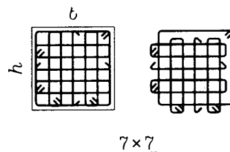
芯柱 XZ 配筋构造
