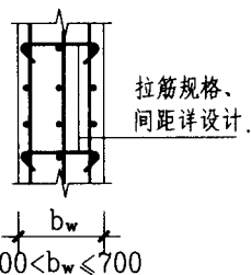
剪力墙三排配筋
