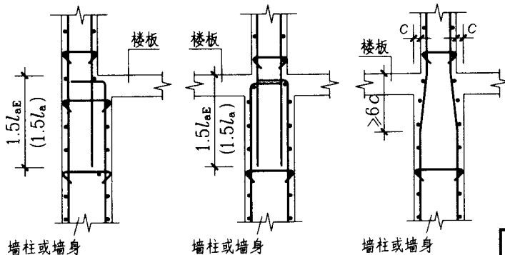
剪力墙变截面处竖向分布钢筋构造
