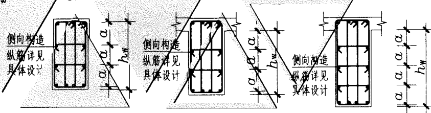
梁侧面纵向构造筋和拉筋
