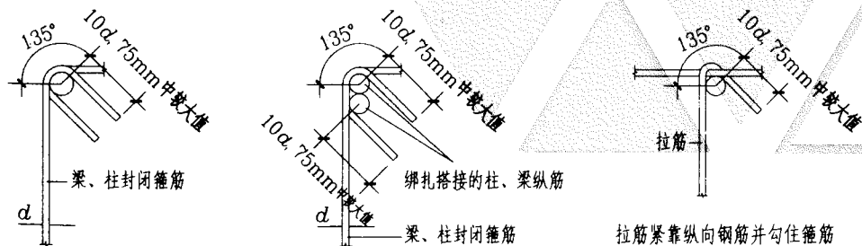
梁、柱、剪力墙箍筋和拉筋弯钩构造
