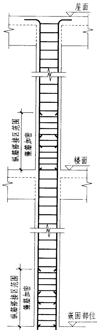
非抗震 KZ 箍筋构造
