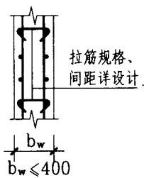
剪力墙双排配筋
