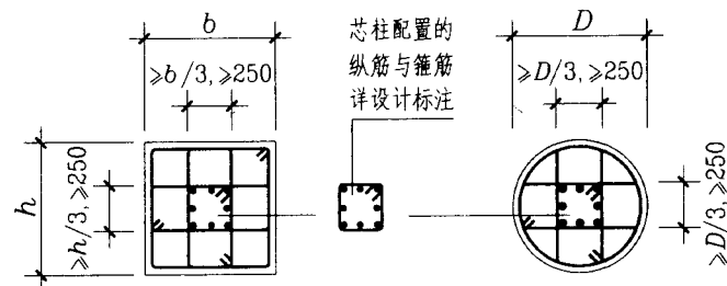
芯柱 XZ 配筋构造
