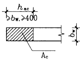
构造边缘暗柱 GAZ
