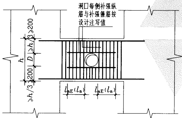
连梁中部圆形洞口补强钢筋构造
