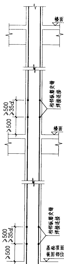
焊接连接
