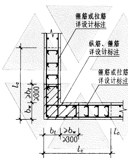
约束边缘转角墙 (柱) YJZ
