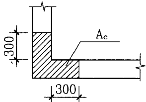
构造边缘转角墙 (柱) GJZ
