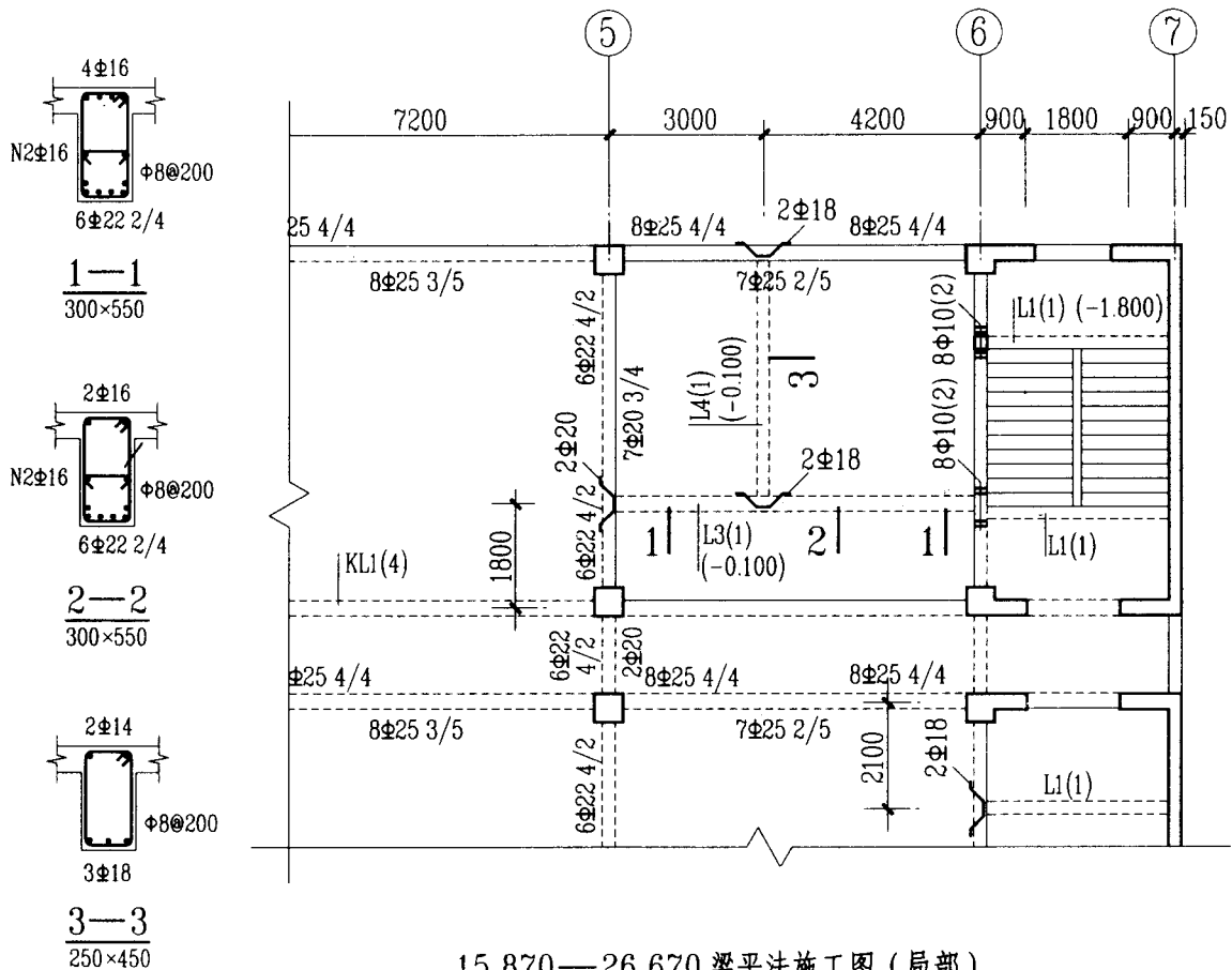
图 4.3.5 梁平法施工图截面注写方式示例
