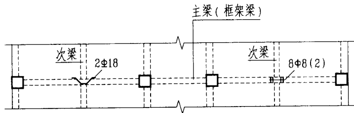
图 4.2.4b 附加箍筋和吊筋的画法示例
