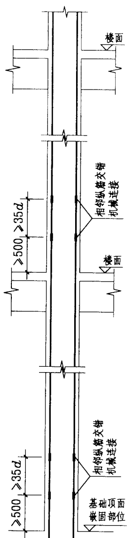
机械连接
