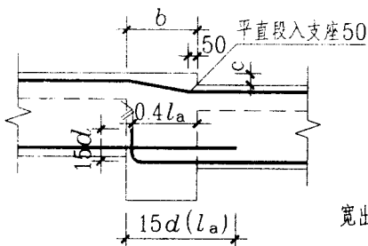
② c/(b-50) \leq 1/6 时, 上部纵筋连续布置。
