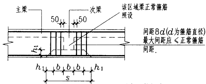
附加箍筋构造
