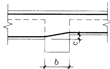
④ c/b \leq 1/6 时, 支座两边相同直径的下部纵筋可连续布置。
