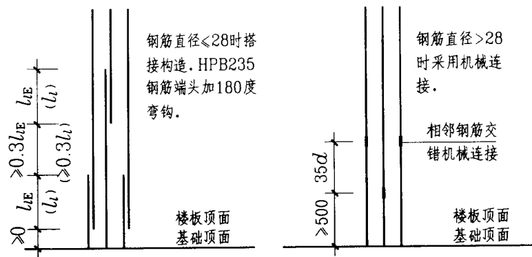
构造边缘构件纵向钢筋连接构造
