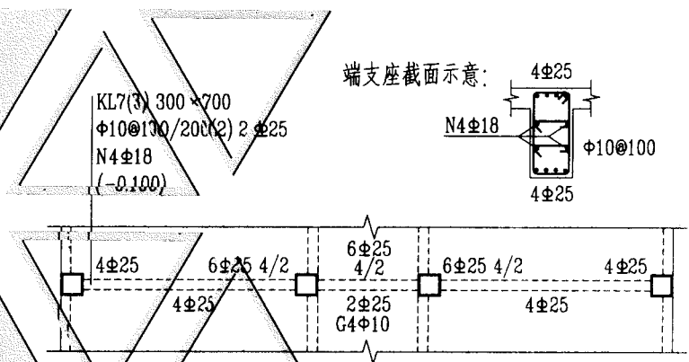
图 4.2.4a 大小跨梁的注写示例
