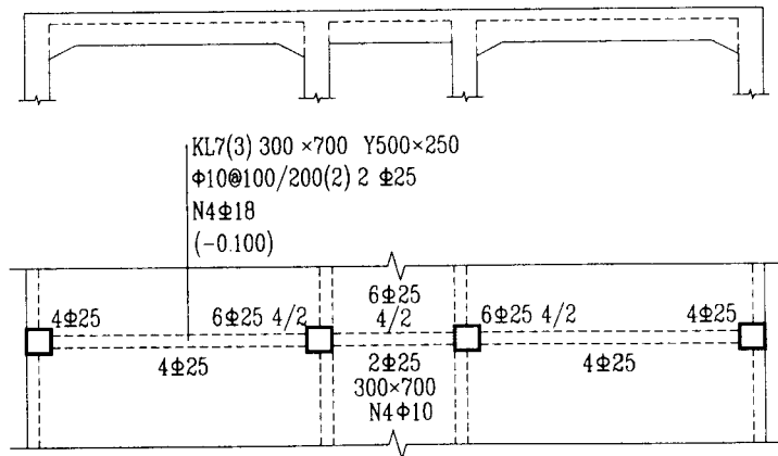
图 4.2.4c 梁加腋平面注写方式表达示例
