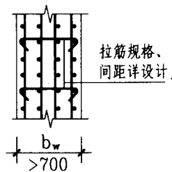
剪力墙四排配筋
