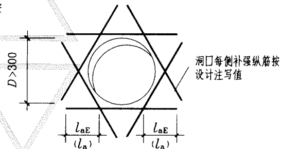
剪力墙圆形洞口直径 大于300时补强纵筋构造
