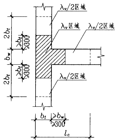
约束边缘翼墙 (柱) YYZ
