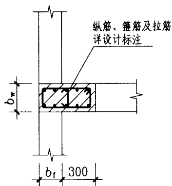
构造边缘翼墙(柱) GYZ
