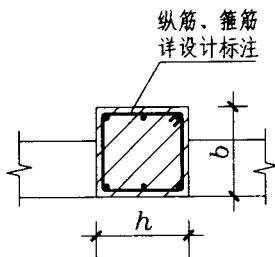
扶壁柱 FBZ
