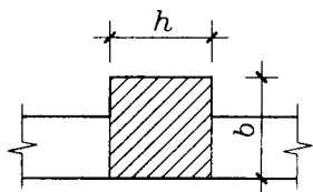
约束边缘翼墙 (柱) YYZ
