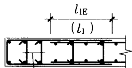
双列拉筋
