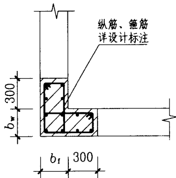
构造边缘转角墙(柱) GJZ
