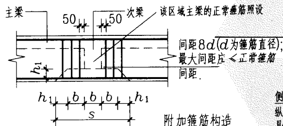
非框架梁 L 配筋构造 (括号内的数字用于弧形非框架梁)
