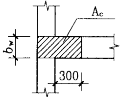
构造边缘翼墙 (柱) GYZ
