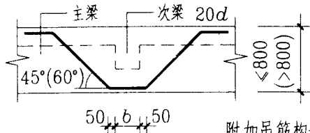
附加吊筋构造
