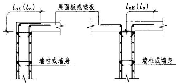
剪力墙竖向钢筋顶部构造
