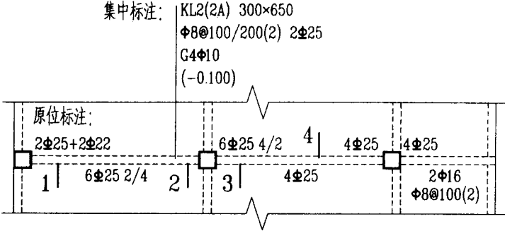
图 4.2.1 平面注写方式示例
