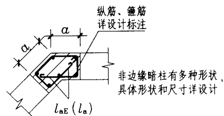
非边缘暗柱 AZ
