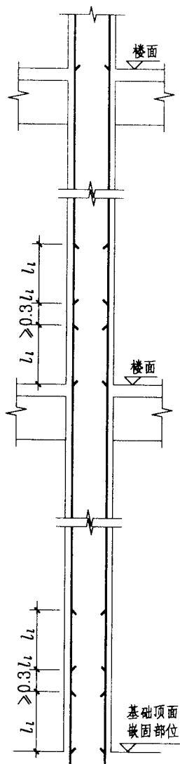
绑扎搭接
