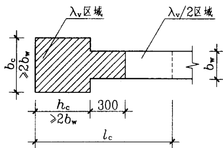
约束边缘端柱 YDZ
