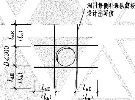
剪力墙圆形洞口直径 不大于300时补强纵筋构造
