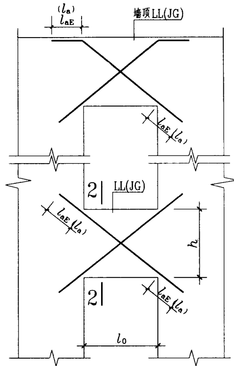
连梁斜向交叉钢筋构造
