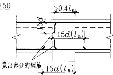
③ 当支座两边梁宽不同时, 将无法直锚的纵筋弯锚入梁内。或当支座两边纵筋根数不同时, 可将多出的纵筋弯锚入梁内。
