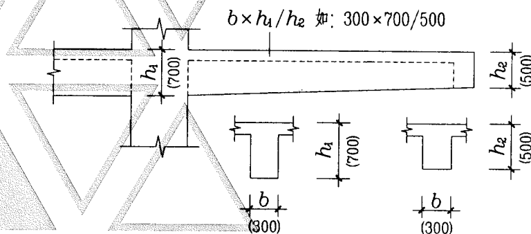
图4.2.3b 悬挑梁不等高截面尺寸注写示意
