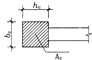
构造边缘端柱 GDZ
