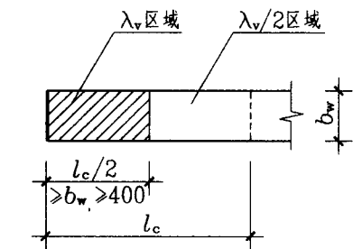
约束边缘暗柱 YAZ
