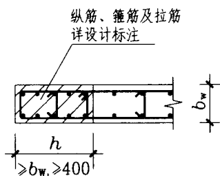
构造边缘暗柱 GAZ
