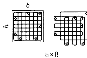
矩形箍筋复合方式
