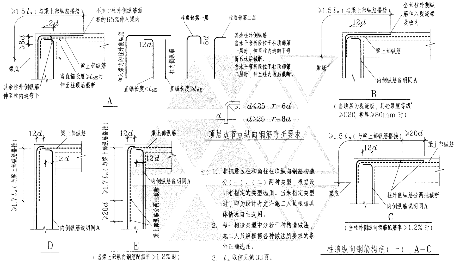
柱顶纵向钢筋构造(二) D、E
