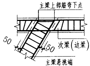
主次梁斜交箍筋构造
