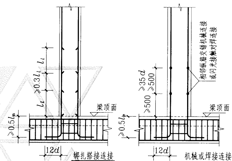
梁上柱 LZ 纵筋构造
