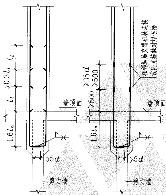
绑扎搭接连接
