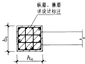
构造边缘端柱 GDZ
