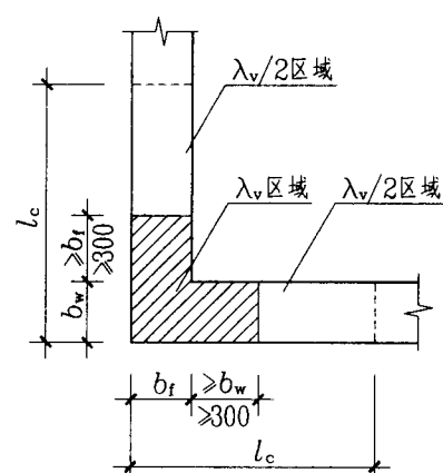
约束边缘转角墙 (柱) YJZ
