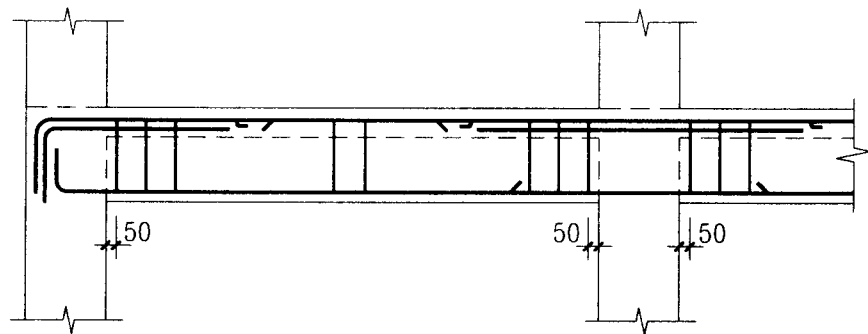
非抗震框架梁KL、WKL
