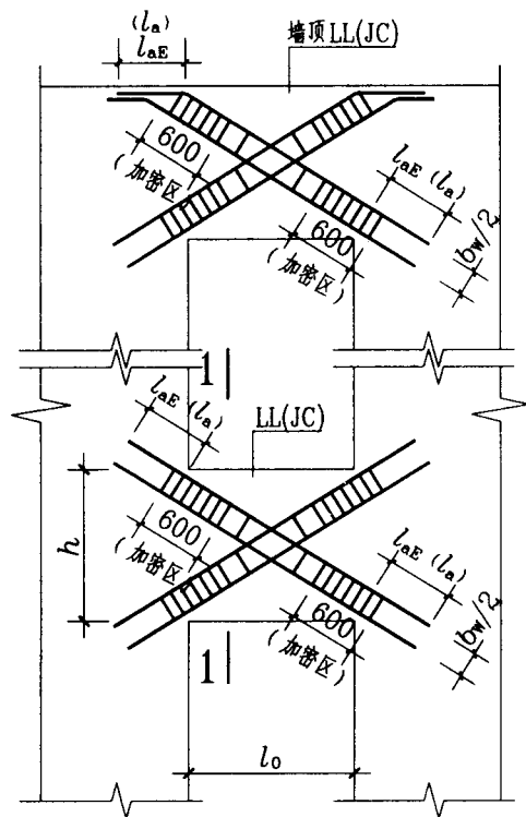
连梁斜向交叉暗撑构造
