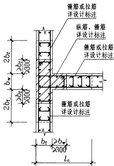
约束边缘翼墙 (柱) YYZ
