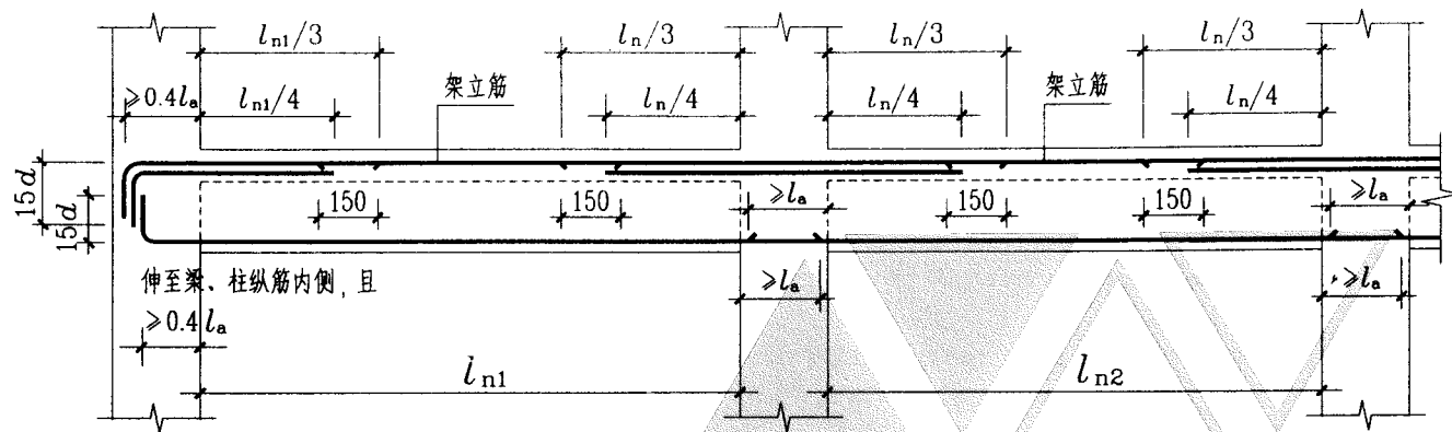
非抗震楼层框架梁 KL (端支座弯锚)
