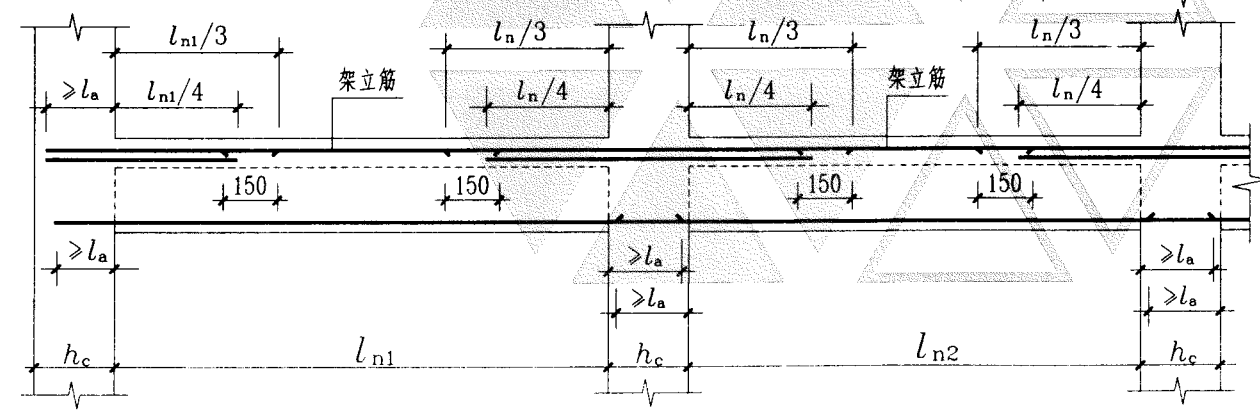
非抗震楼层框架梁 KL (端支座直锚)
