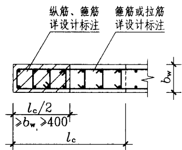
约束边缘暗柱 YAZ
