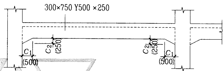
图4.2.3a 加腋梁截面尺寸注写示意
